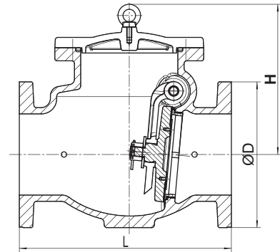
Size 5"-12"
